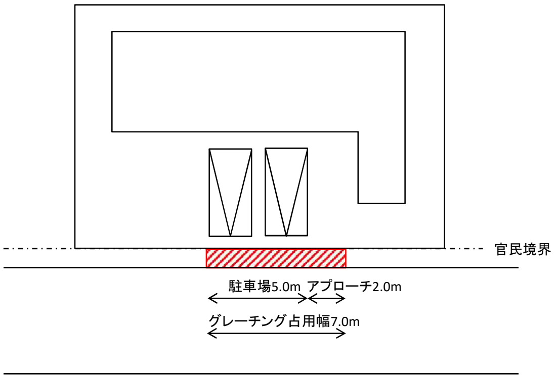
平面図
