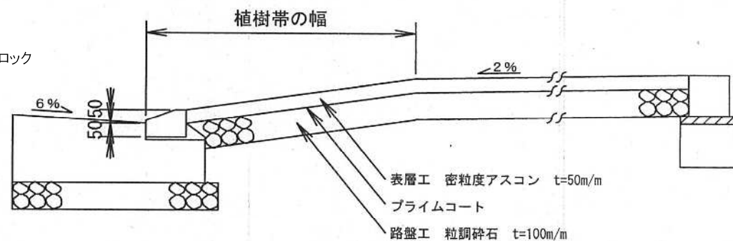
A-A' 断面図
