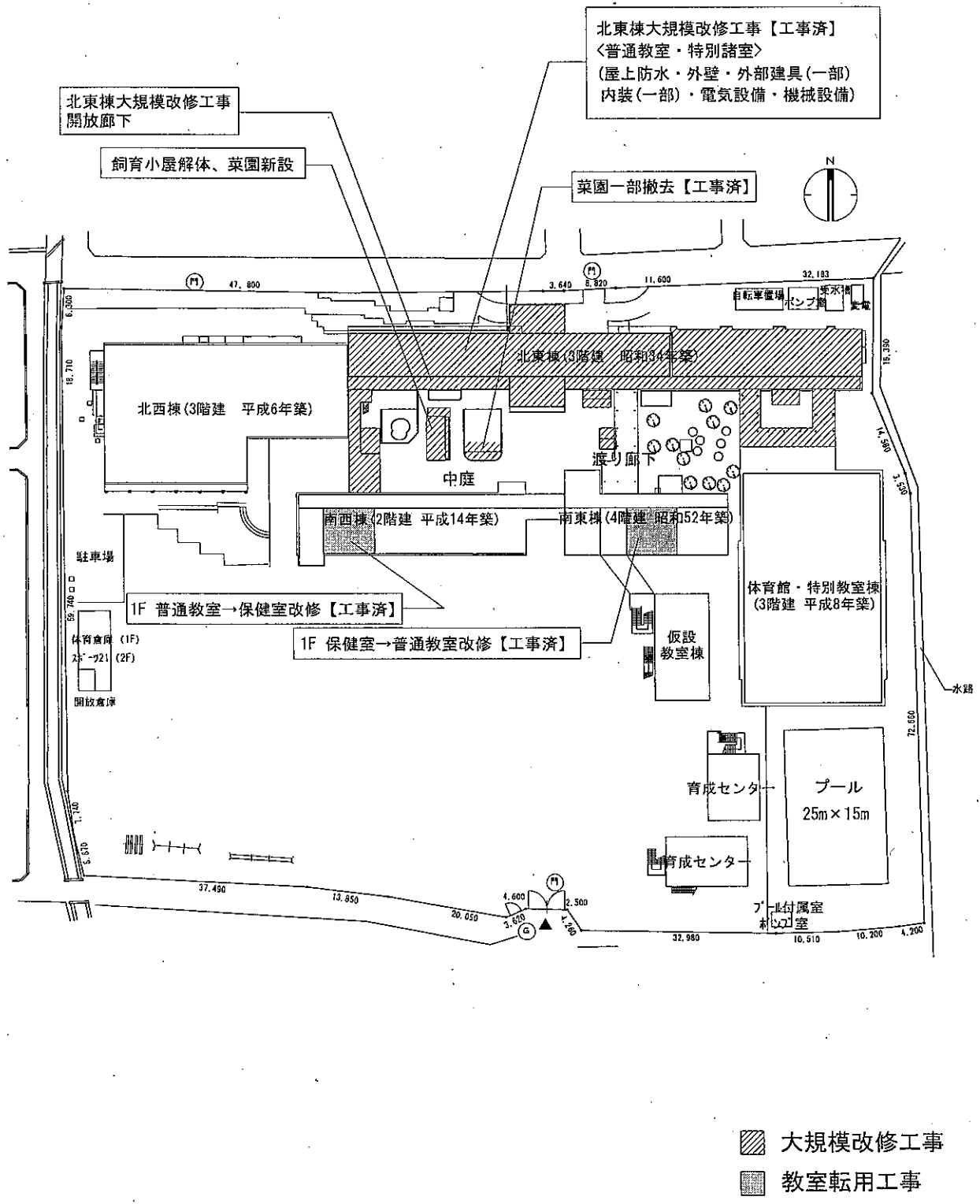
甲東小学校北東棟大規模改修工事 配置図(1/1000)
