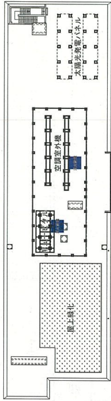
屋根伏図
