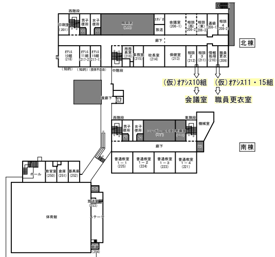
【変更前】2階 平面図
