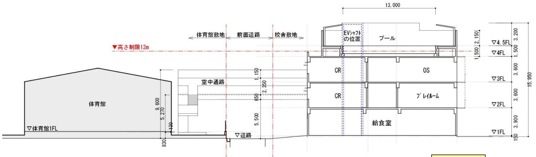
断面図
