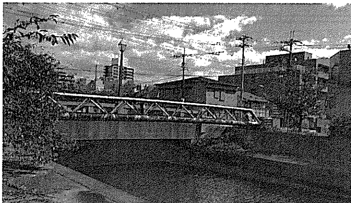
甲子園網引町の新川水管橋。トラス型の補剛形式を採用している
